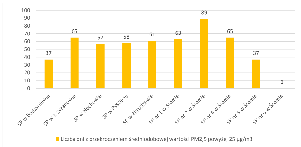
Rysunek 15 Liczba dni z przekroczeniem średniodobowej wartości PM2,5 powyżej 25 µg/m3, źródło: dane Urzędu Miejskiego w Śremie
