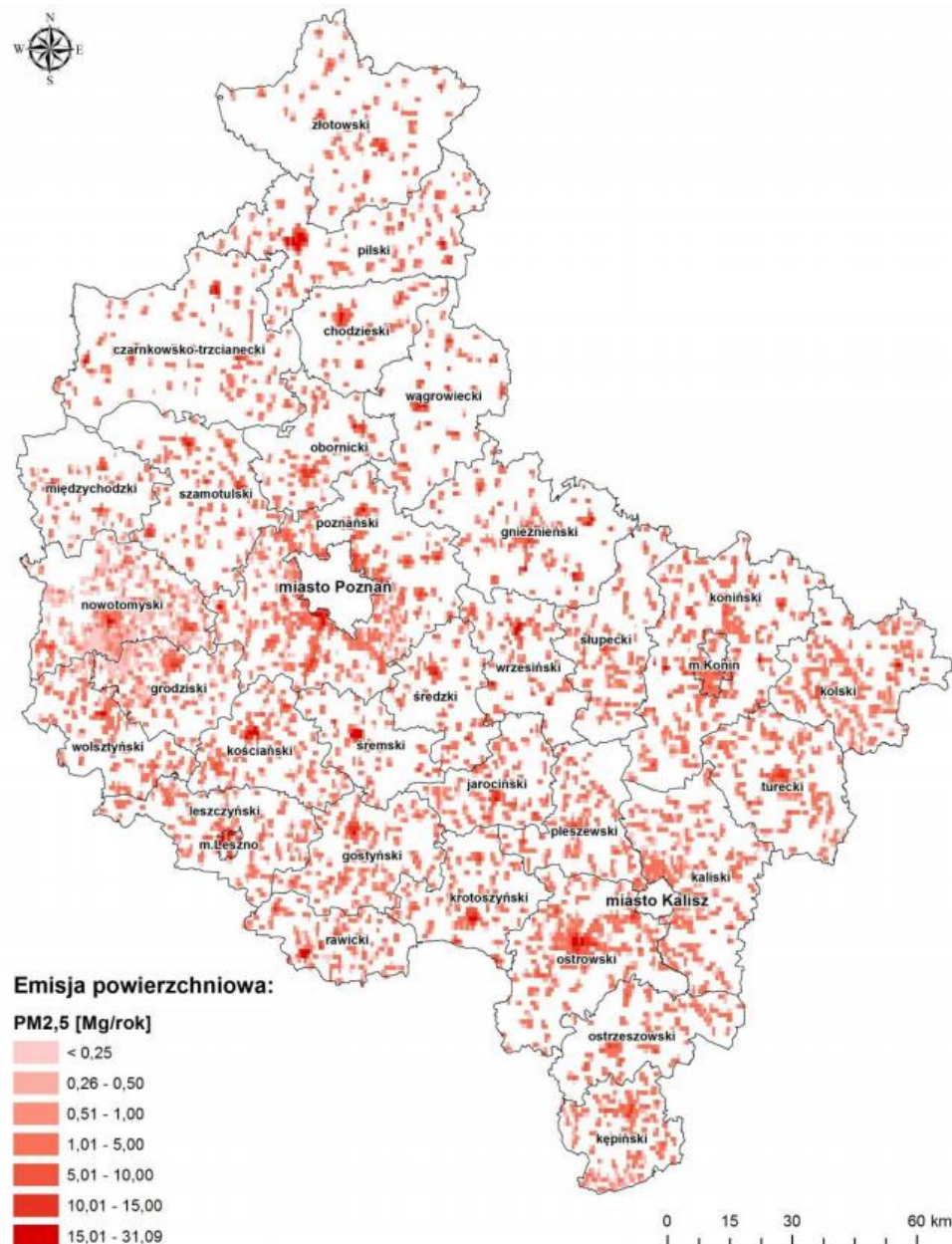
Rysunek 4 Lokalizacja i wielkość emisji pyłu PM 2,5 ze źródeł powierzchniowych na terenie strefy wielkopolskiej; źródło: Program ochrony powietrza dla strefy wielkopolskiej w zakresie pyłu PM 10 , PM 2,5 oraz B(a)P
